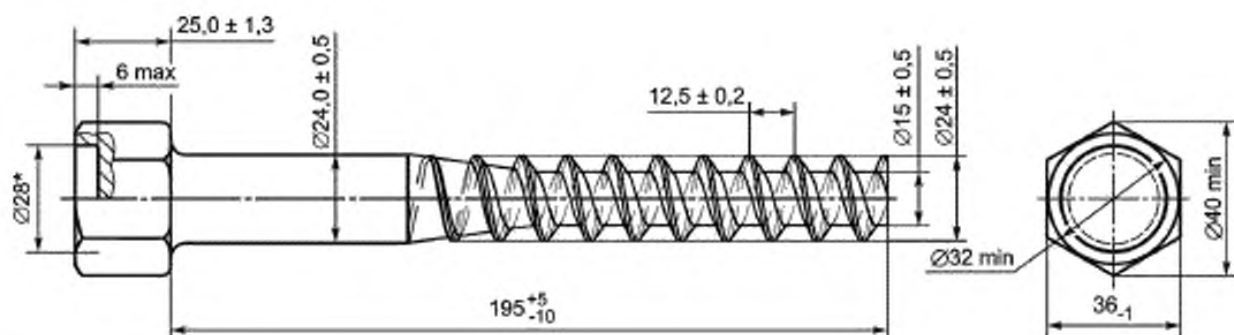
Конструкция Б, исполнение 2
