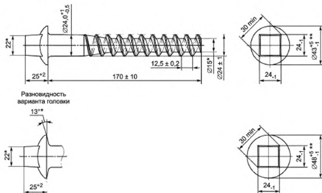
Конструкция А, исполнение 1
